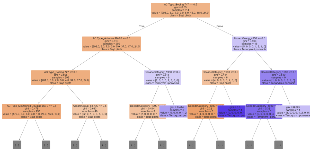
Uprozczone drzewo klasyfikacyjne dla CauseCategory
